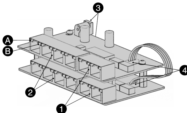
Figur 4. PoE switch med ekstrakort
