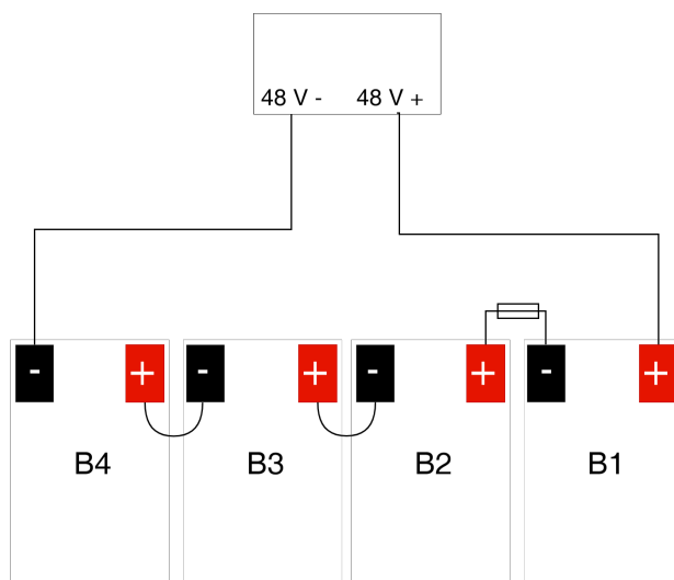
Figur 2. Kopplingschema för batterier i batteribackup
